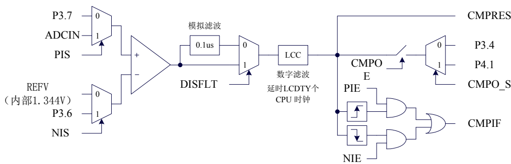
比较器内部结构
