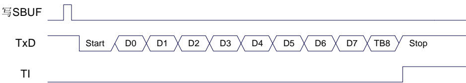
发送数据（串口1模式3）
