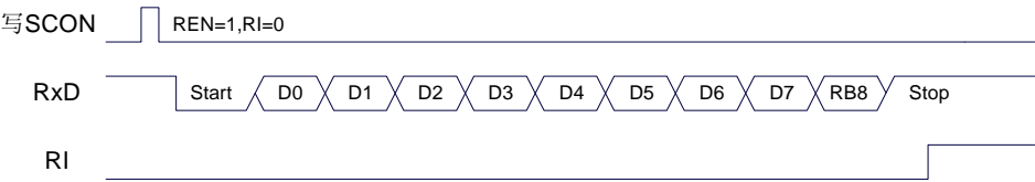
接收数据（串口1模式3）
