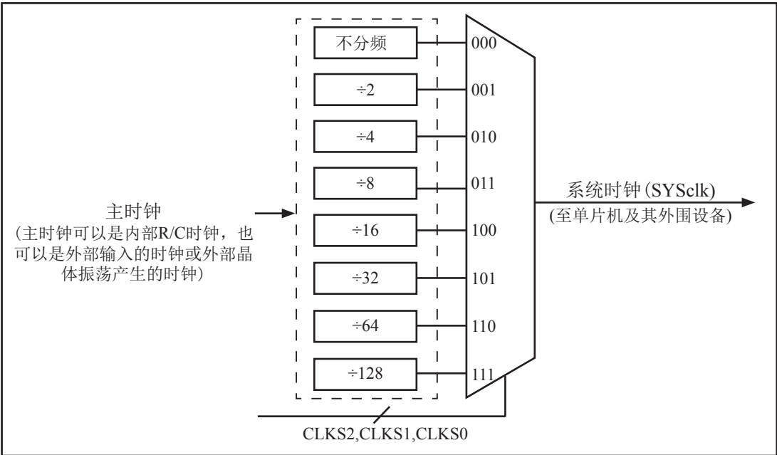
时钟结构
